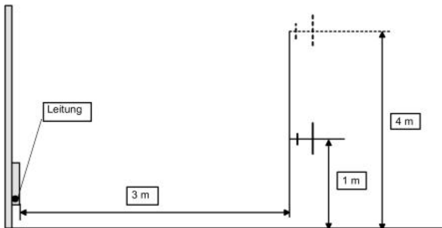
Bild 2: Höhenscan der Antenne
