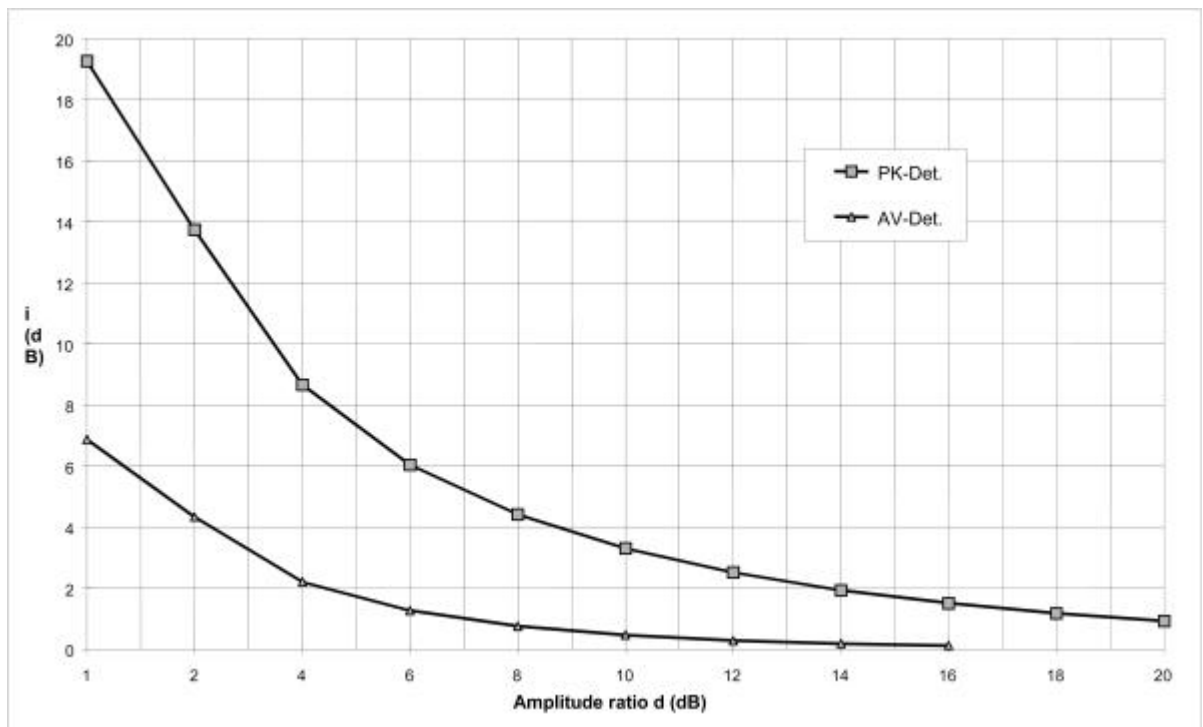
Bild A.4.1 Bestimmung der Amplitude des Störsignals mittels des Amplitudenverhältnisses \mathbf{d} und des Faktors \mathbf{i}
