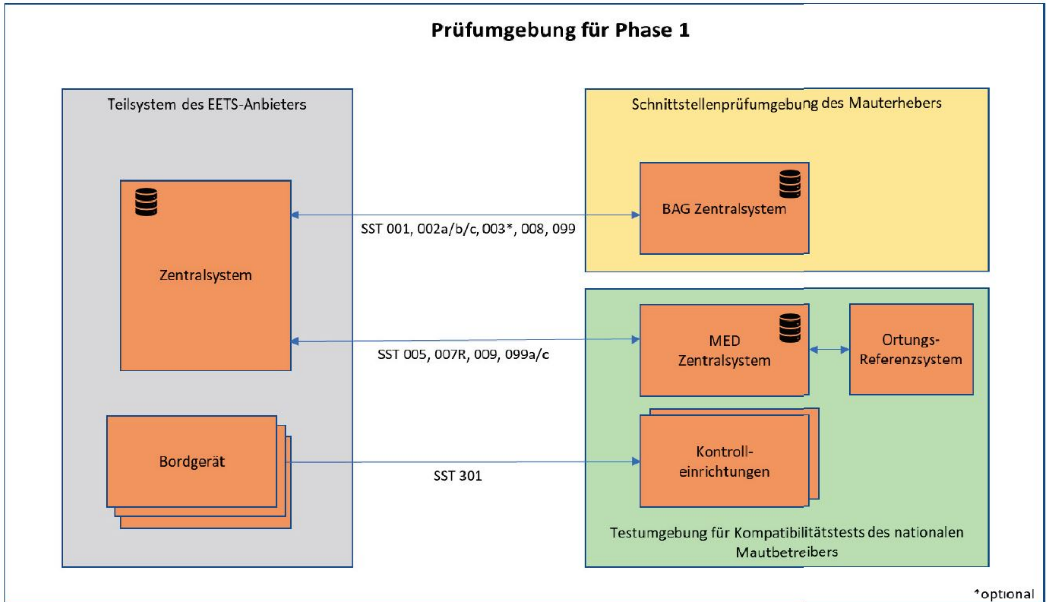
Abbildung 2: Testumgebung Phase 1
